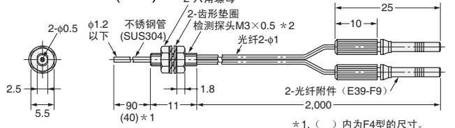
E32-DC200FR(F4R)
