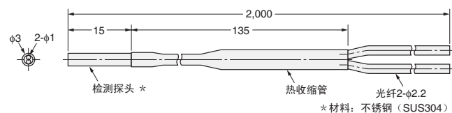
E32-D12R
