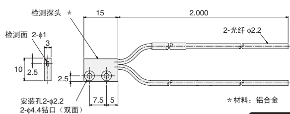
E32-D15XR
