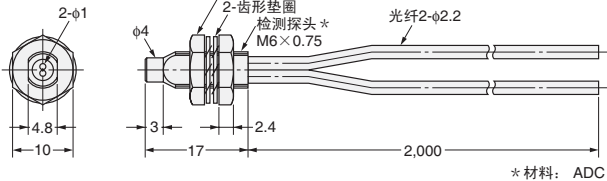
E32-D11R
