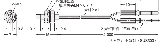
E32-D211R
