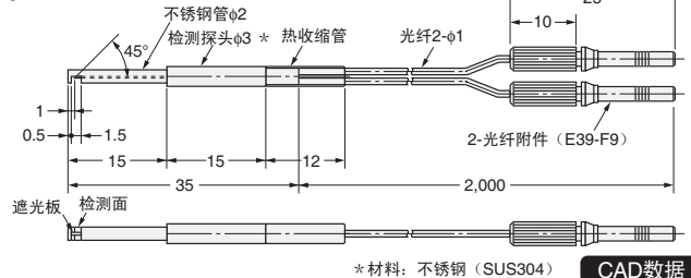
E32-D24R
