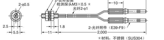
E32-D21R
