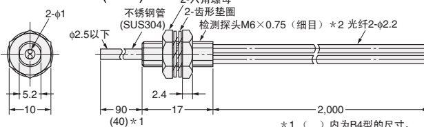
E32-DC200BR(B4R)
