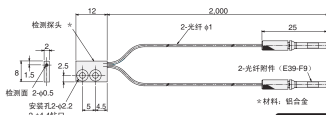
E32-D25XR
