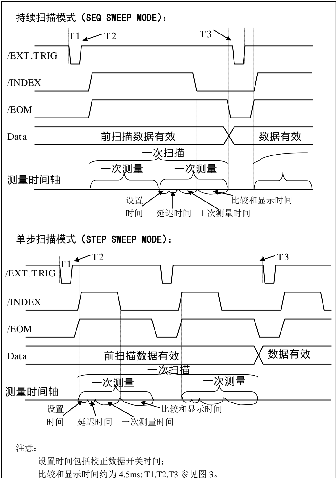
图 5 计时图解
