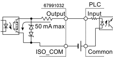
PLC 的 PN 输入
