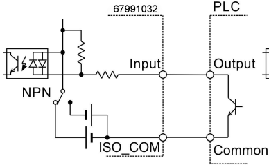
PLC 的 NPN 输出
