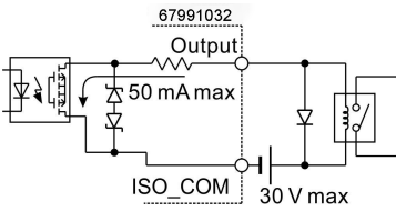
驱动继电器
