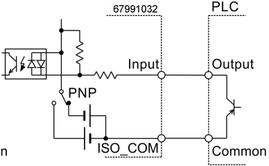
PLC 的 PNP 输出
