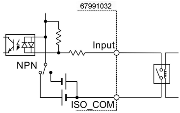
继电器输入
