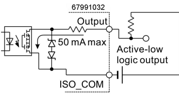
逻辑电平输出
